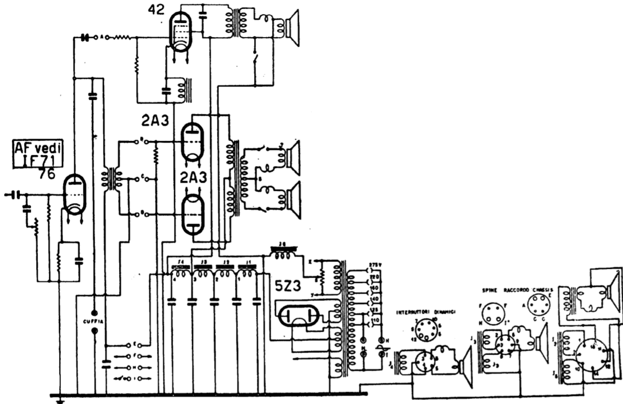
Schemi delle BF dei ricevitori IMCA-RADIO mod. « IF 103 »
